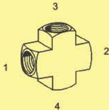
BP-5652 - Cross (1) (2) (3) (4) Fem. Pipe
