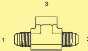
BJ-2602 - Tee (1) (2) Male 37° (3) Fem. Pipe
