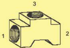
BIF-652 - Tee (1) (2) Fem. Inv. Flare (3) Fem. Pipe
