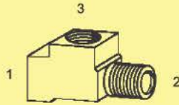
BIF-752 - Tee (1) (3) Fem. Inv. Flare (2) Male Pipe
