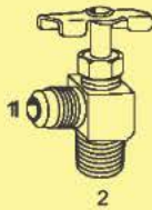
BNV-101F - 90° (1) Male 45° Flare (2) Male Pipe
