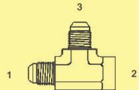
BJ-2606 - Tee (1) (3) Male 37° (2) Fem. Pipe
