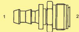
SPO-2290 - Str. (1) Hose Barb (2) Male Inv. Flare Swivel
