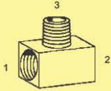
BIF-602 - Tee (1) (2) Fem. Inv. Flare (3) Male Pipe
