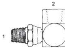
5502-S - 90° (1) Male Pipe Swivel (2) Fem. Pipe
