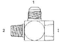
2613 - Tee
