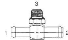
4606-NWO - Tee
