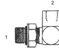
6805-NWO - 90° (1) Adj. O Ring (2) Fem. Pipe
