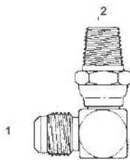
2501-S - 90°
