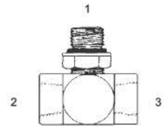
6870-NWO - Tee (1) Adj. O Ring (2) (3) Fem. O Ring
