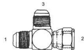
6602 - Tee
