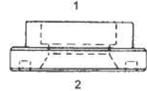
SF-3300-62 (1) (2) Braze Flange Code 62
