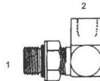
6815-NWO - 90° (1) Adj. O Ring (2) Fem. O Ring
