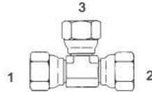
Y-6606-F - Tee (1) (2) (3) 37° Fem. Swivel
