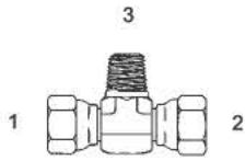
Y-6603-F - Tee (1) (2) 37° Fem. Swivel (3) Male Pipe
