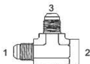
Y-2606-F - Tee (1) (3) Male 37° (2) Fem. Pipe
