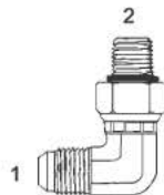
Y-6801-F-S-O - 90°
