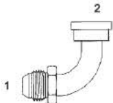
Y-1704-62 - 90° (1) Male 37° (2) O Ring Flange Code 62
