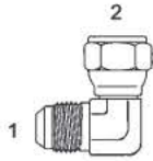
Y-6500-F - 90° (1) Male 37° (2) 37° Fem. Swivel
