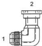
Y-1704-F-62 - 90° (1) Male 37° (2) O Ring Flange Code 62
