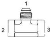
Y-2612-F - Tee (1) Male 37° (2) (3) Fem. Pipe
