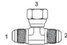
Y-6600-F - Tee (1) (2) Male 37° (3) 37° Fem. Swivel
